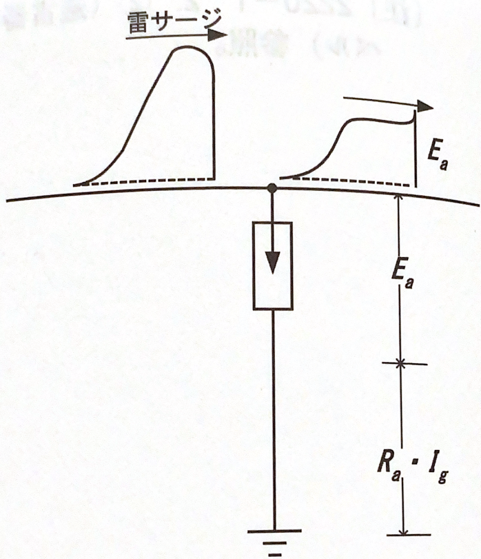
2220-1図 避雷器による雷サージ抑制効果
